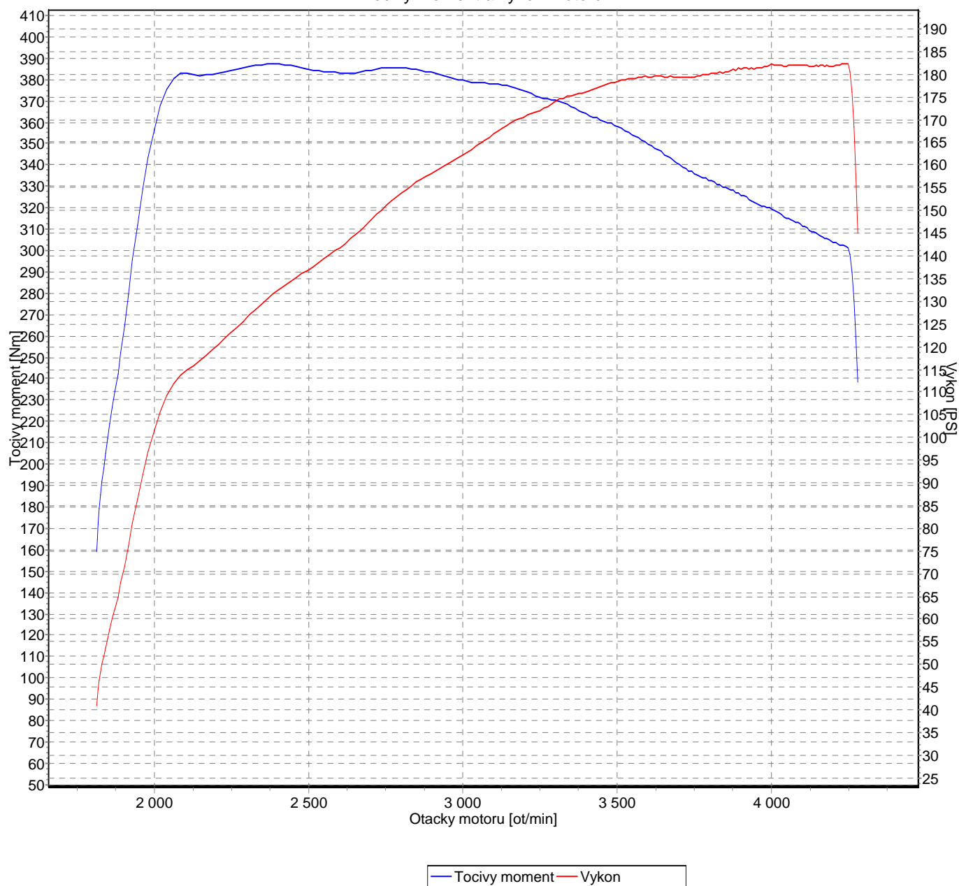
Tocivy moment a výkon motoru
