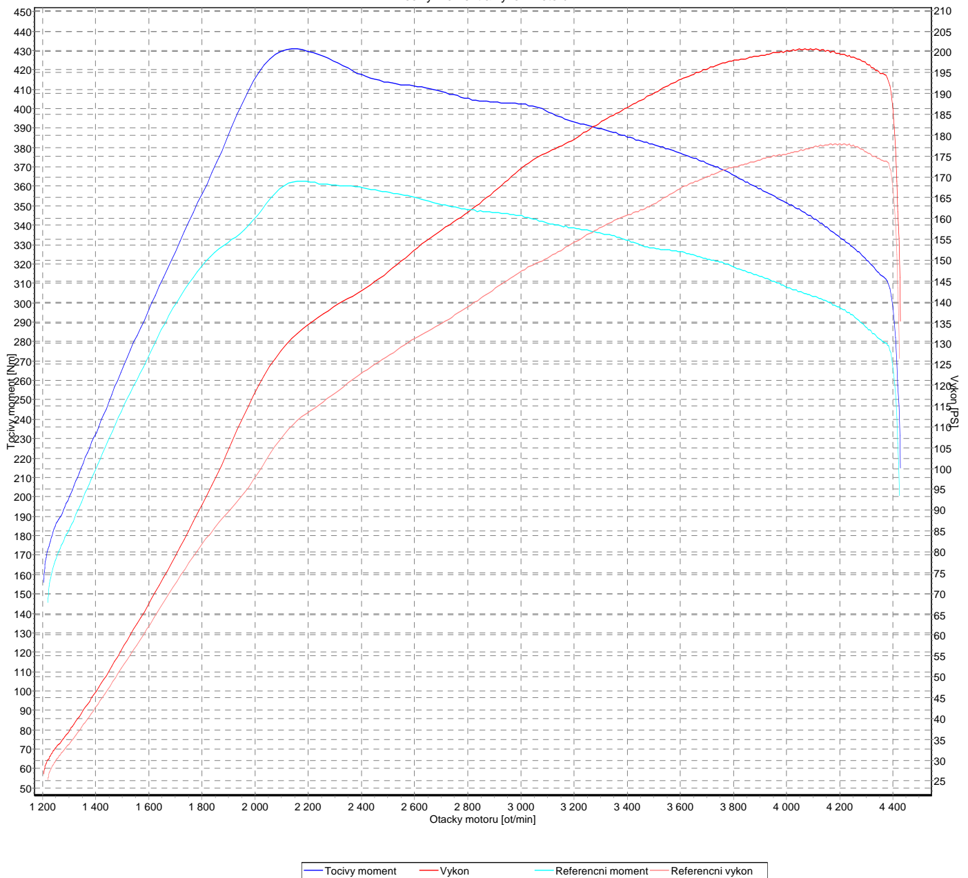
Tocivy moment a vykon motoru
